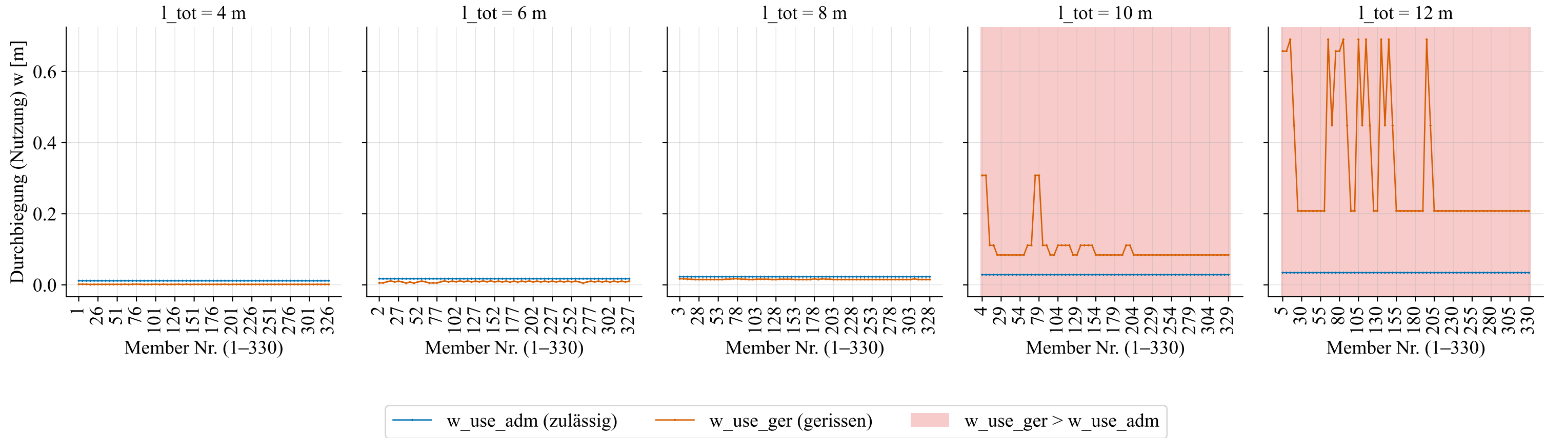
Durchbiegung w_{\text{use\_adm}} (zulässig) vs. w_{\text{use\_ger}} (gerissen) je Member, kategorisiert nach Spannweite (Members_rc_rib_simple_V3)
